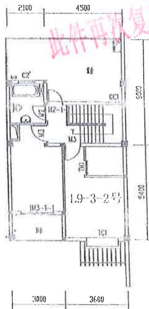
三层平面图
