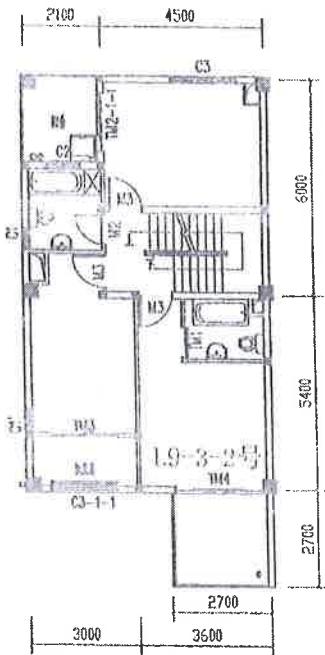
二层平面图
