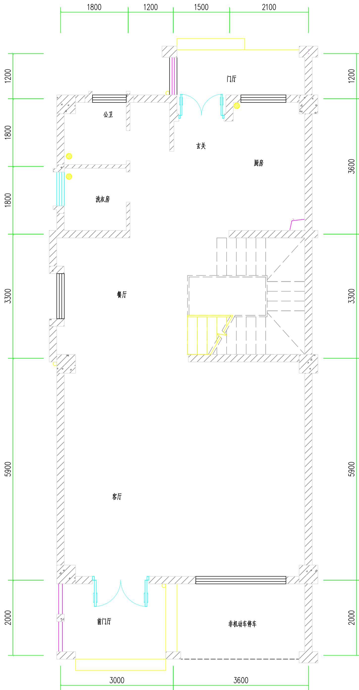
13-1栋一层户型平面图
