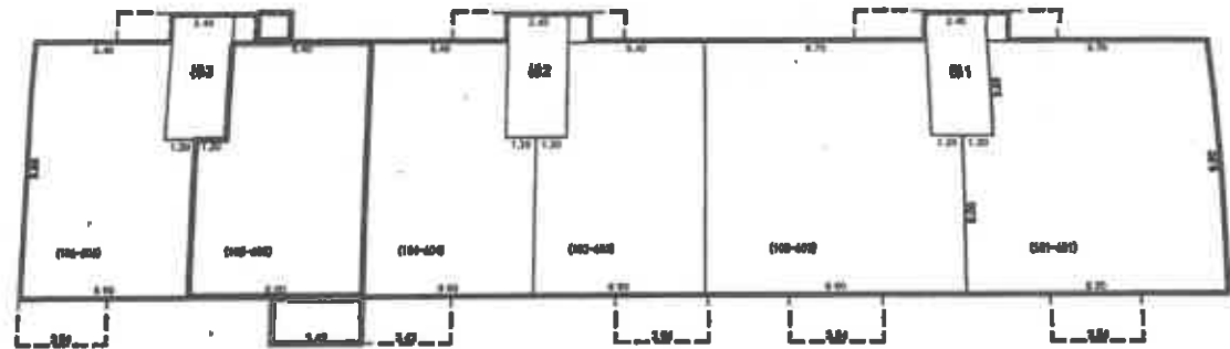
一至六层平面图
