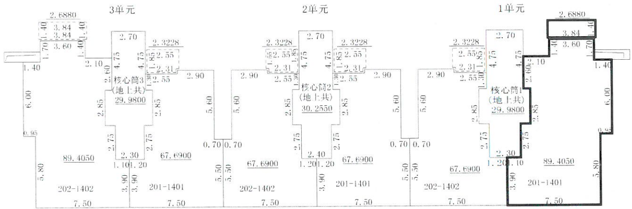
二至十四层平面图
