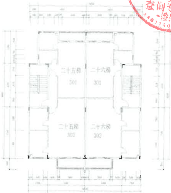
三层平面图
