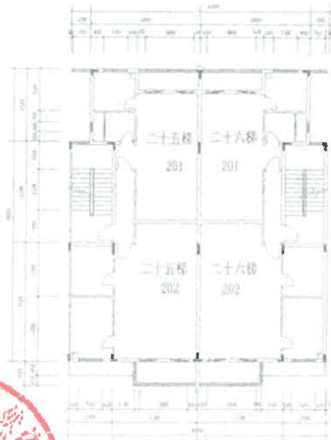
二层平面图
