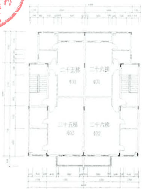
四层平面图
