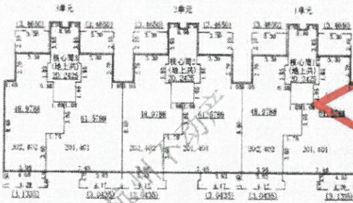
二、四层平面图
