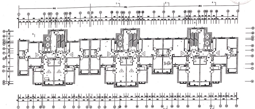
和汇百合湾13#楼三至二十八层平面图
