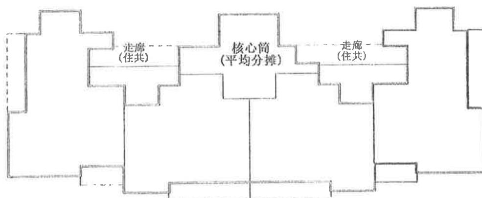
三至十五层平面图
