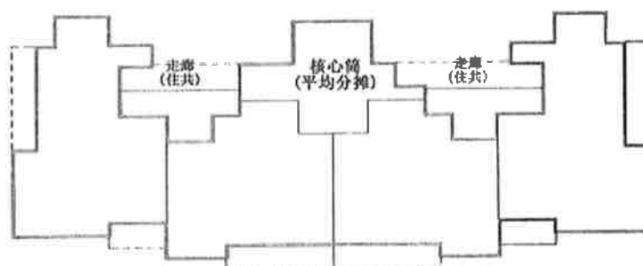
三至十五层平面图
