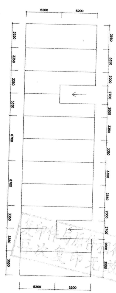
溪美街 一层平面图
