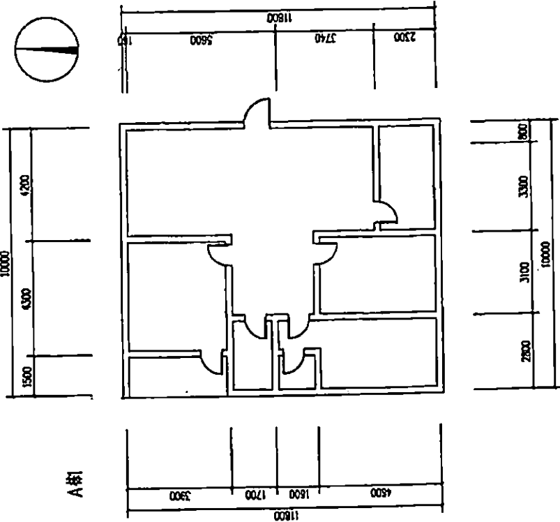
平面图
