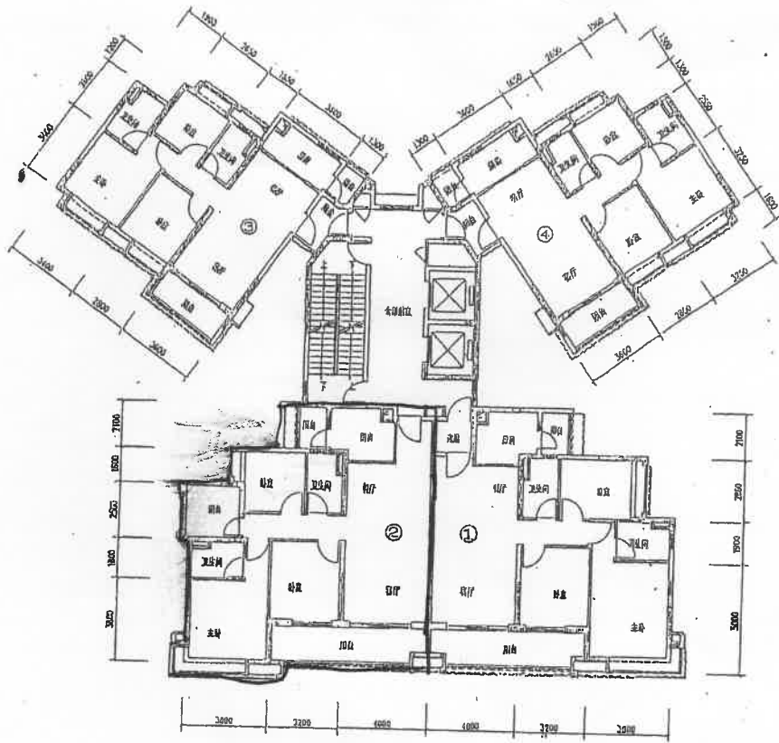
自編5#樓六至二十二層平面图
