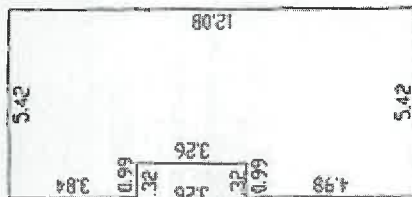
三层平面图
