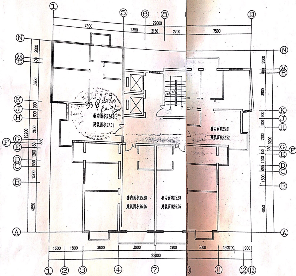
4号楼A单元2-18层平面图
