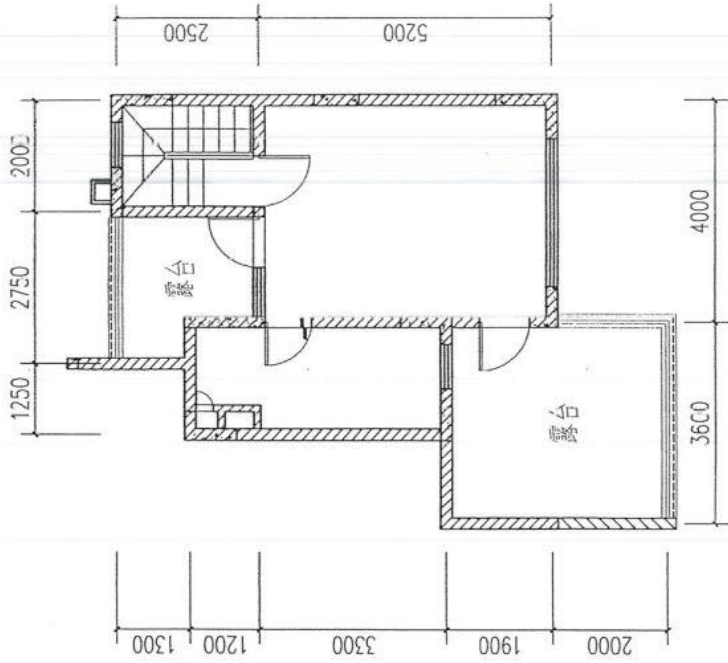
二层平面图
